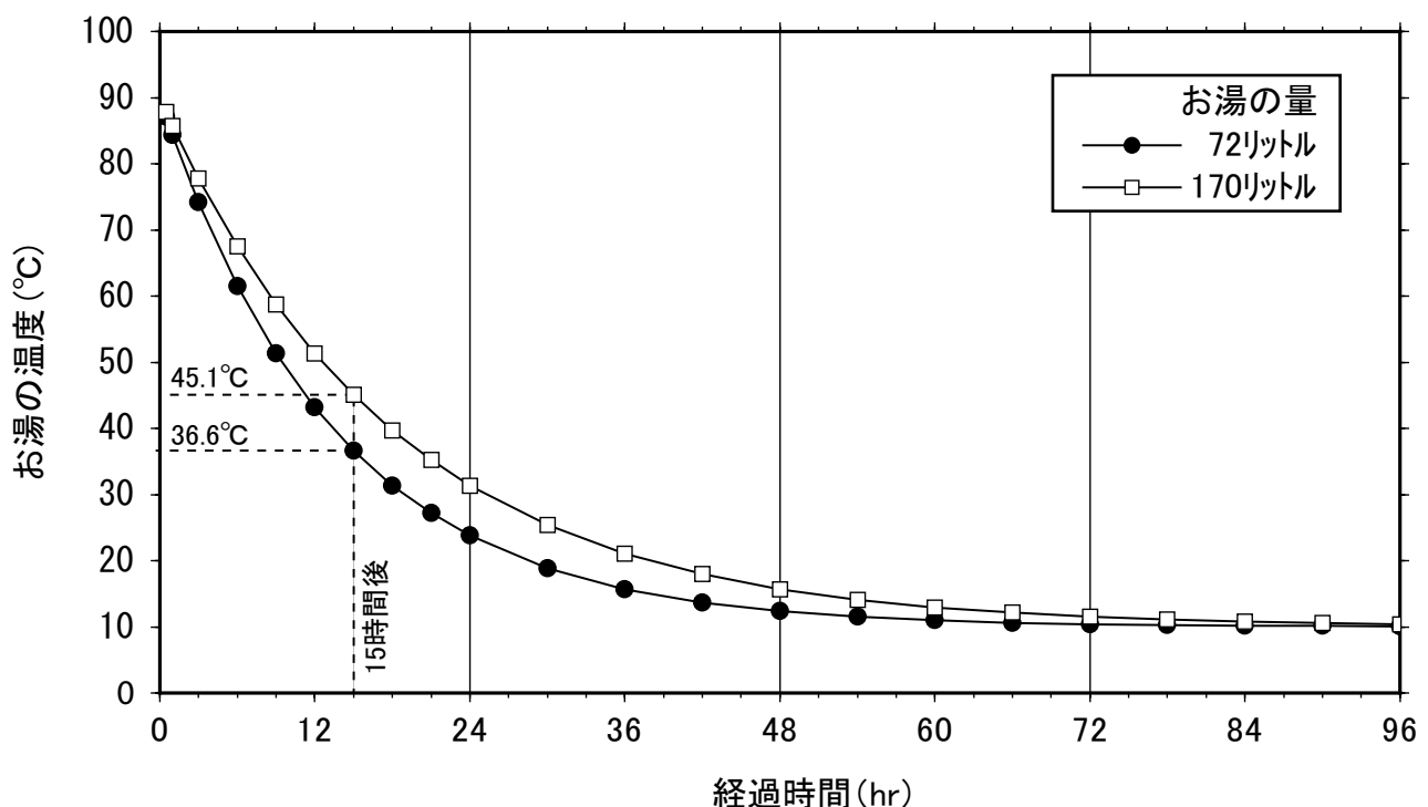
図 2 時間経過とお湯の温度の下がり方
